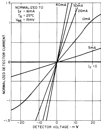
a. LOW LEVEL V-I PLOT
